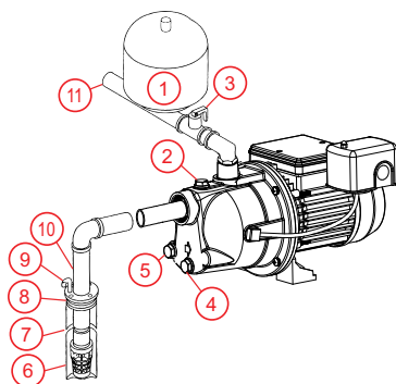
Pozo poco profundo (con válvula de retención en línea)
