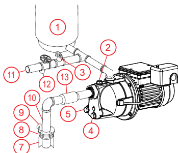
Puits peu profond avec clapet anti-retour en ligne
