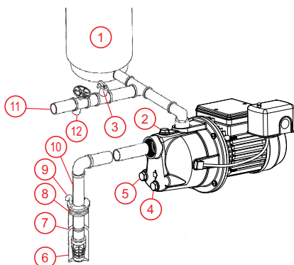
Pozo poco profundo, sistema montado en tanque
