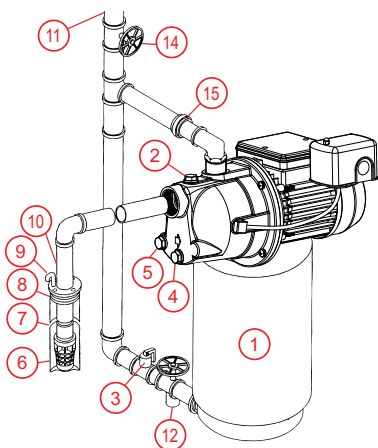
Puits peu profond, système de réservoir monté
