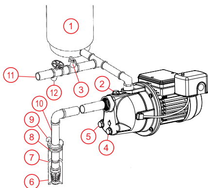
Puits peu profond, système de réservoir monté
