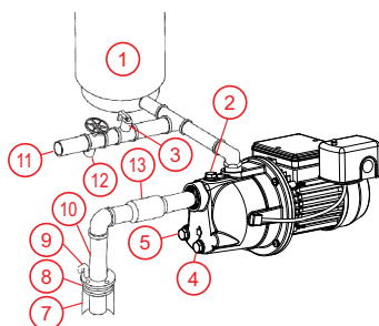
Pozo poco profundo (con válvula de retención en línea)
