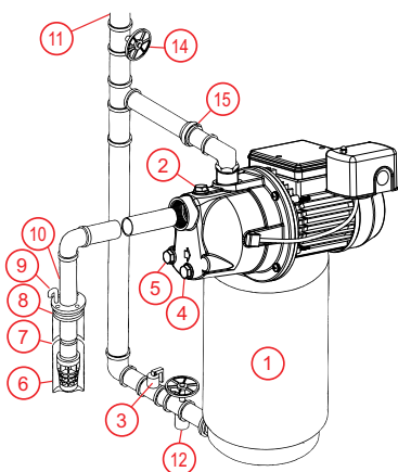
Pozo poco profundo, sistema montado en tanque
