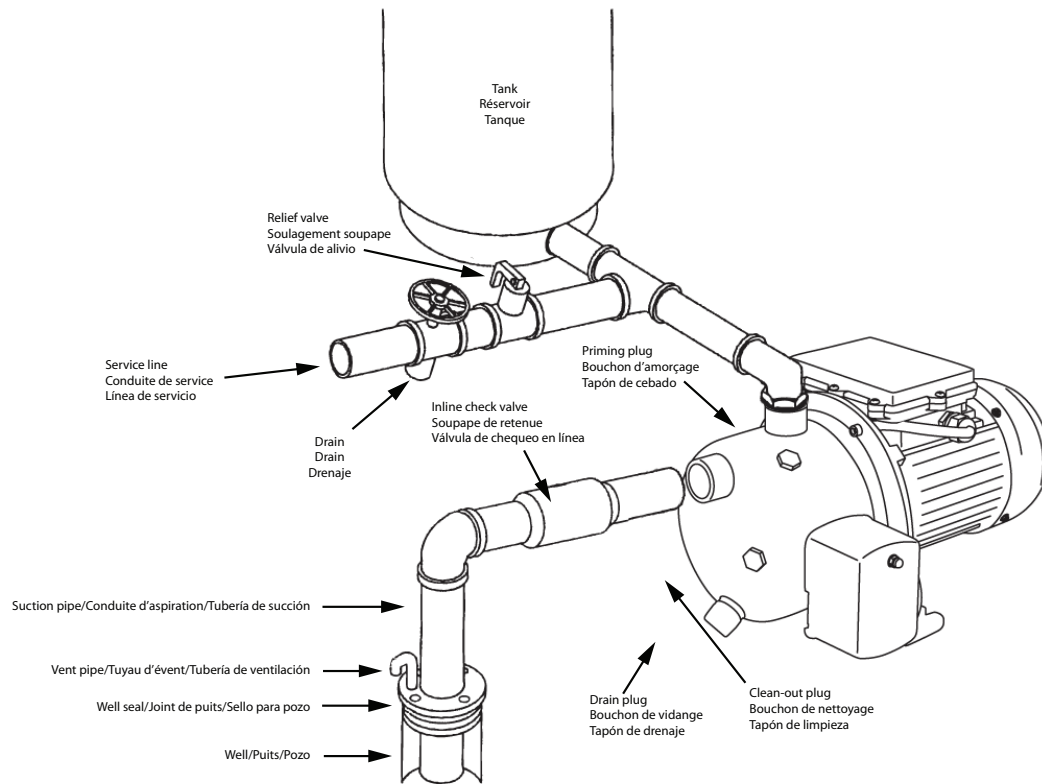
FIGURE 5 SHALLOW WELL (WITH INLINE CHECK VALVE) • PUIS PEU PROFOND (AVEC CLAPET ANTI-RETOUR EN LIGNE) • POZO POCO PROFUNDO (CON VÁLVULA DE RETENCIÓN EN LÍNEA)
