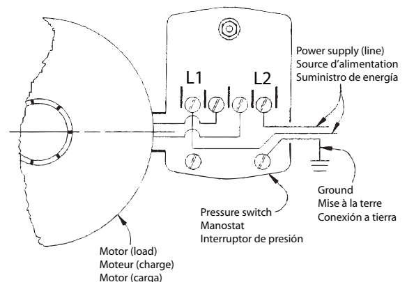
FIGURE 1 ELECTRICAL CONNECTIONS • CONNEXIONS ÉLECTRIQUES • CONEXIONES ELÉCTRICAS
