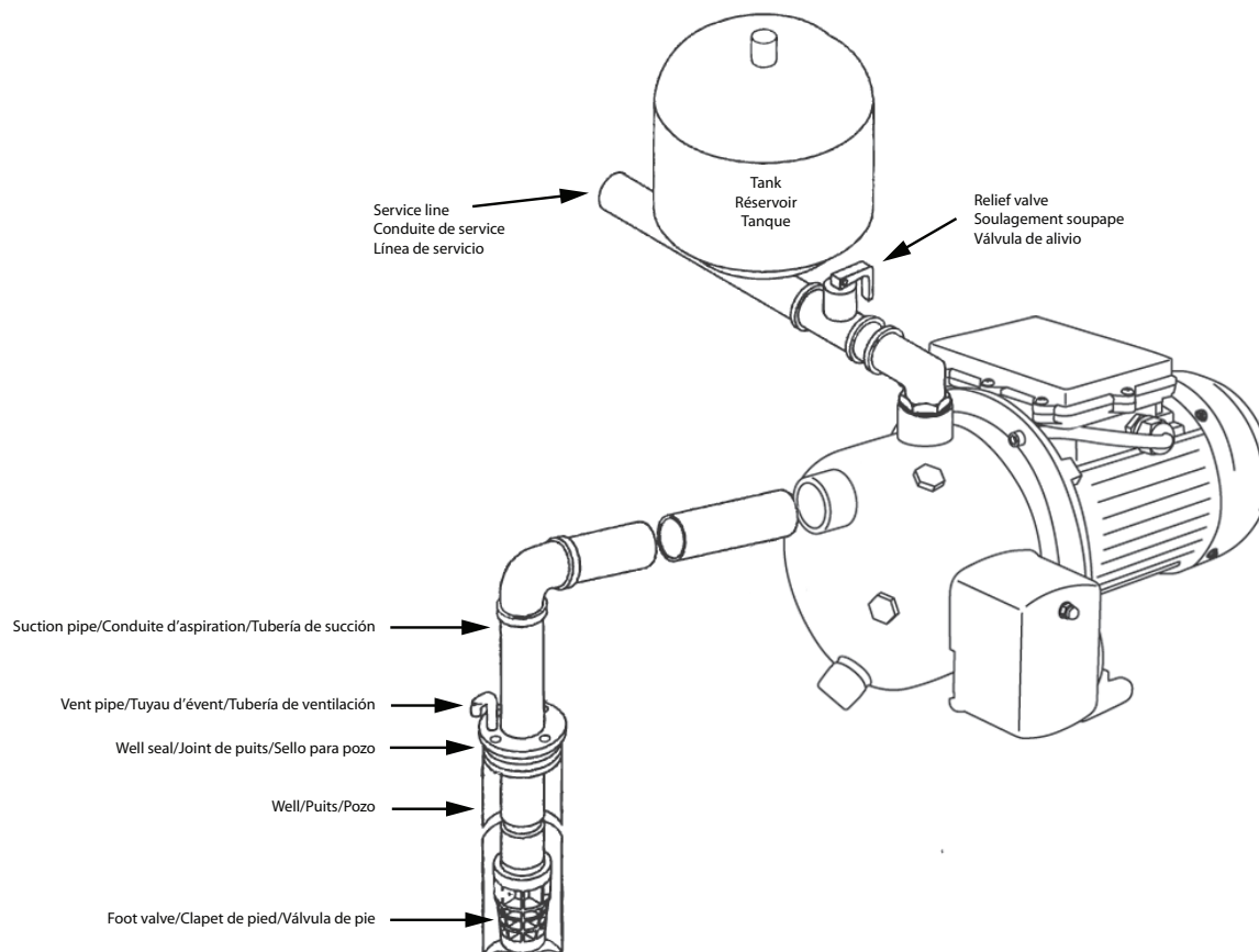
FIGURE 4 SHALLOW WELL - INLINE TANK (WITH FOOT VALVE) • Puits peu profond, réservoir en ligne (avec clapet de pied) • POZO POCO PROFUNDO, TANQUE EN LÍNEA (CON VÁLVULA DE ASPIRACIÓN)
