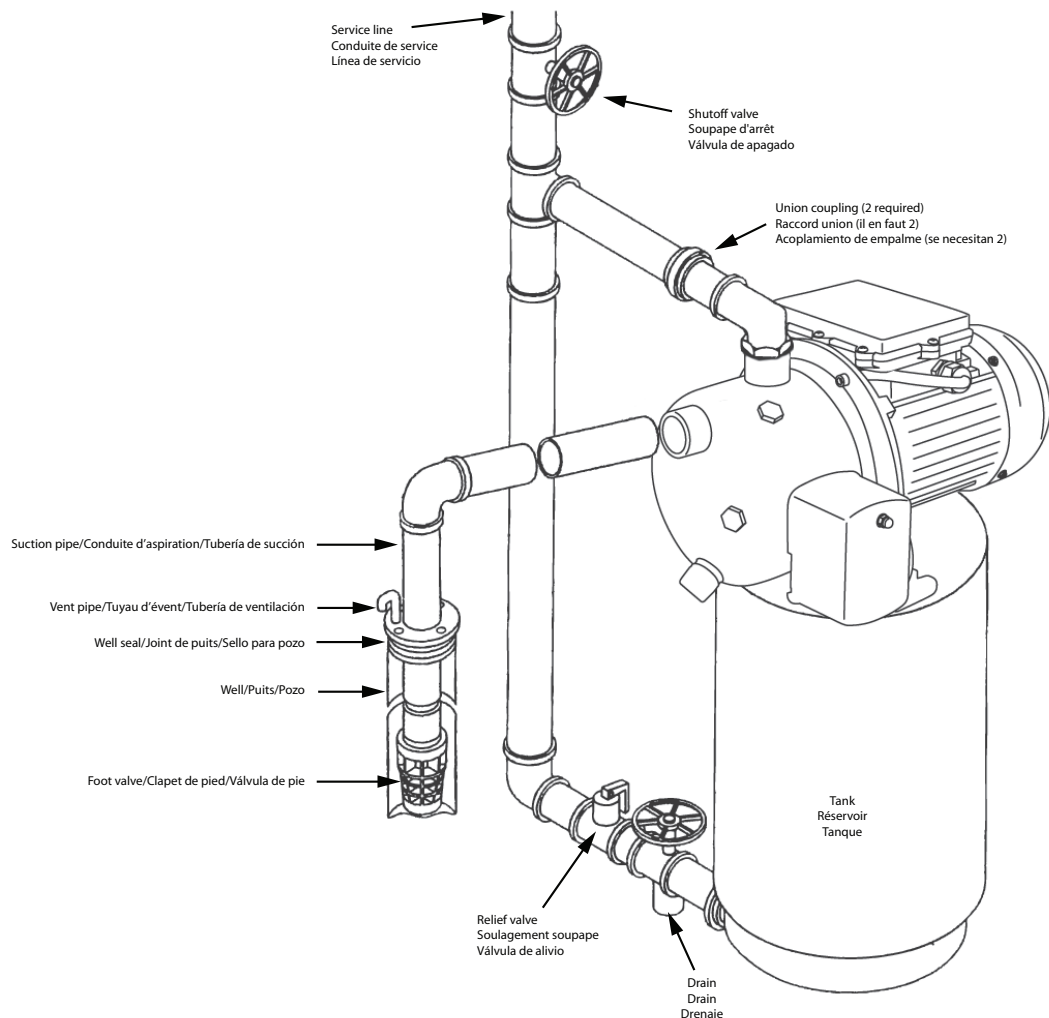
FIGURE 6 SHALLOW WELL - TANK-MOUNTED SYSTEM (WITH FOOT VALVE) • PUIS PEU PROFOND, SYSTÈME DE RÉSERVOIR MONTÉ (AVEC CLAPET DE PIED) • POZO POCO PROFUNDO, SISTEMA MONTADO EN TANQUE (CON VÁLVULA DE ASPIRACIÓN)
