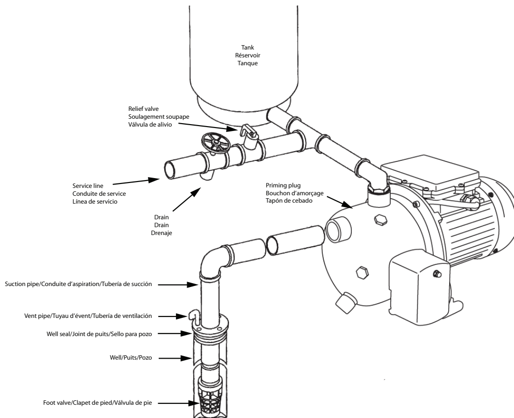
FIGURE 3 SHALLOW WELL (WITH FOOT VALVE) • Puits peu profond (avec clapet de pied) • POZO POCO PROFUNDO (CON VÁLVULA DE ASPIRACIÓN)
